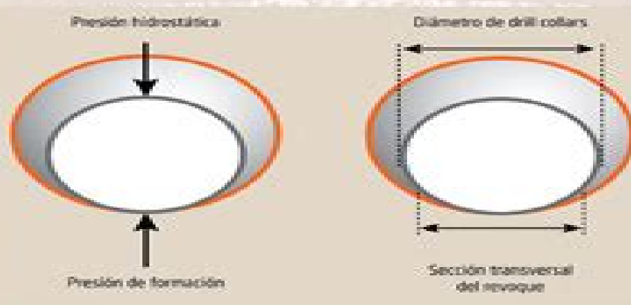
Figura 2. Presión hidrostática y de formación que actúan sobre los drill collars.
