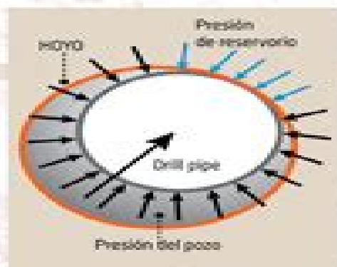
Figura 1. Pega diferencial de tubería.
