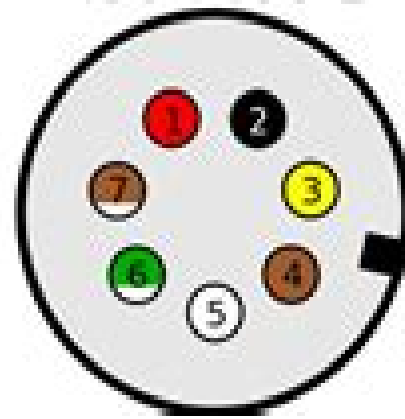
ISO 7638-2
