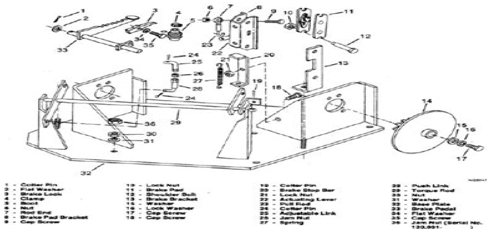
Fig. 1 - Brake
