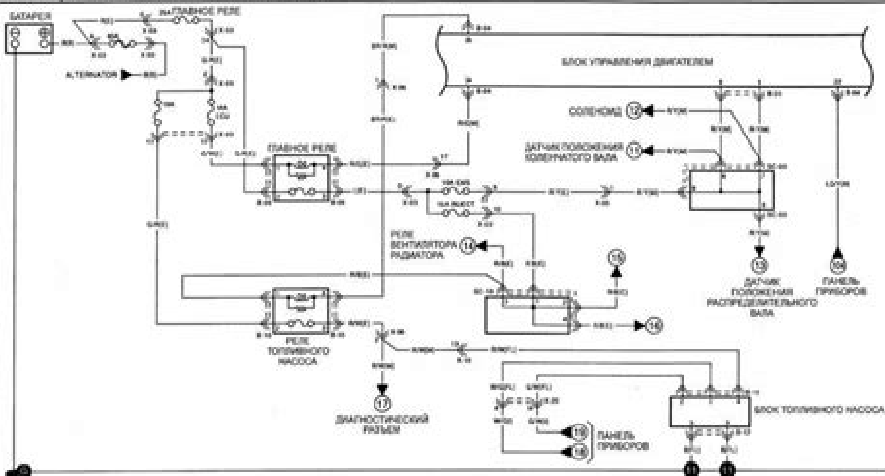
B-1a БЛОК УПРАВЛЕНИЯ ДВИГАТЕЛЕМ
