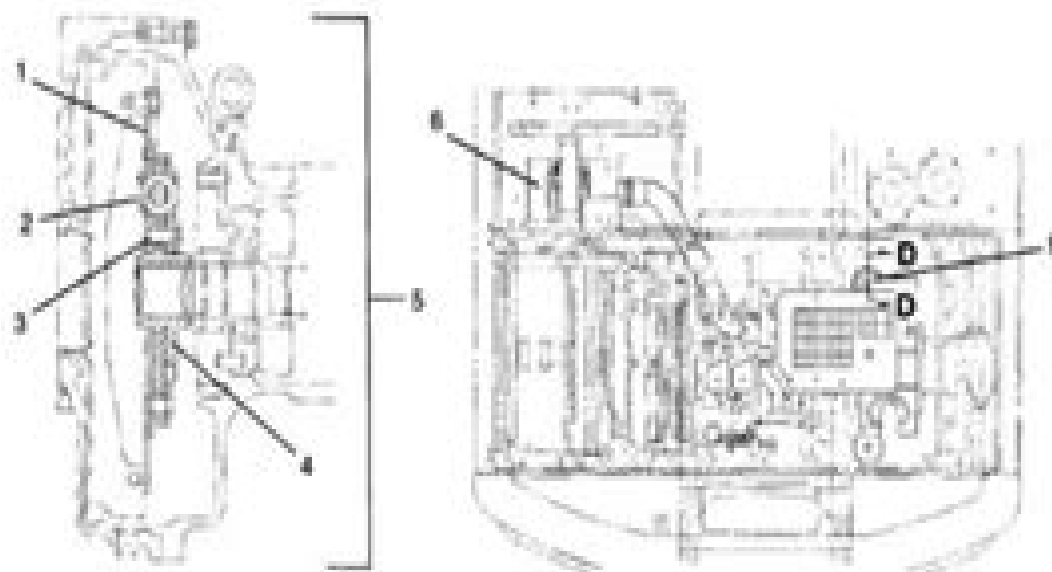
SECTION A-A
