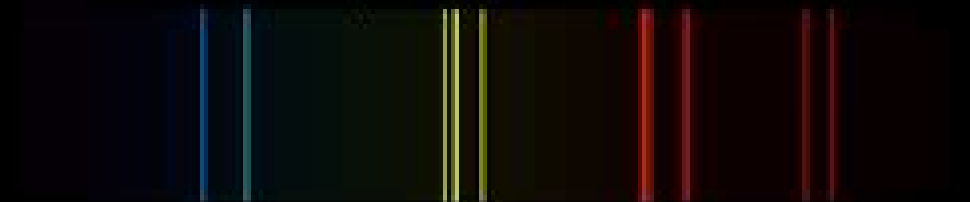
Spectre d'émission
