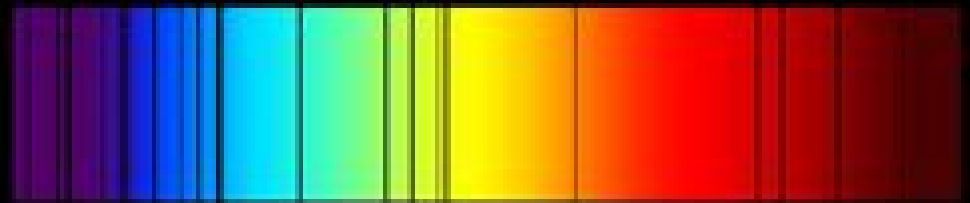
Spectre d'absorption
