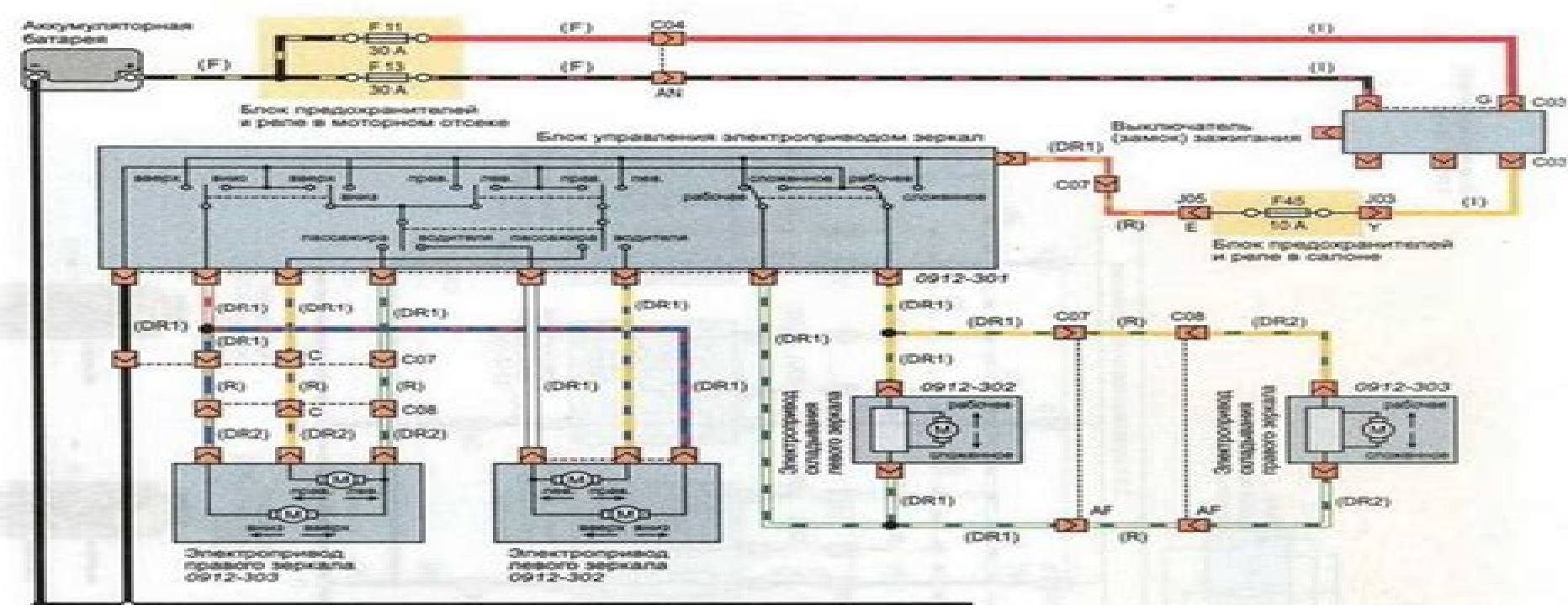
Блок управления электроприводом зеркал (DR1) 0912-301
