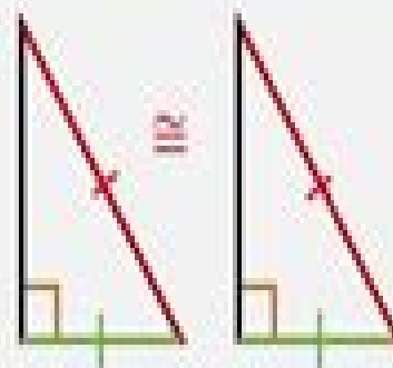
RHL Right-Hypotenuse-Leg
