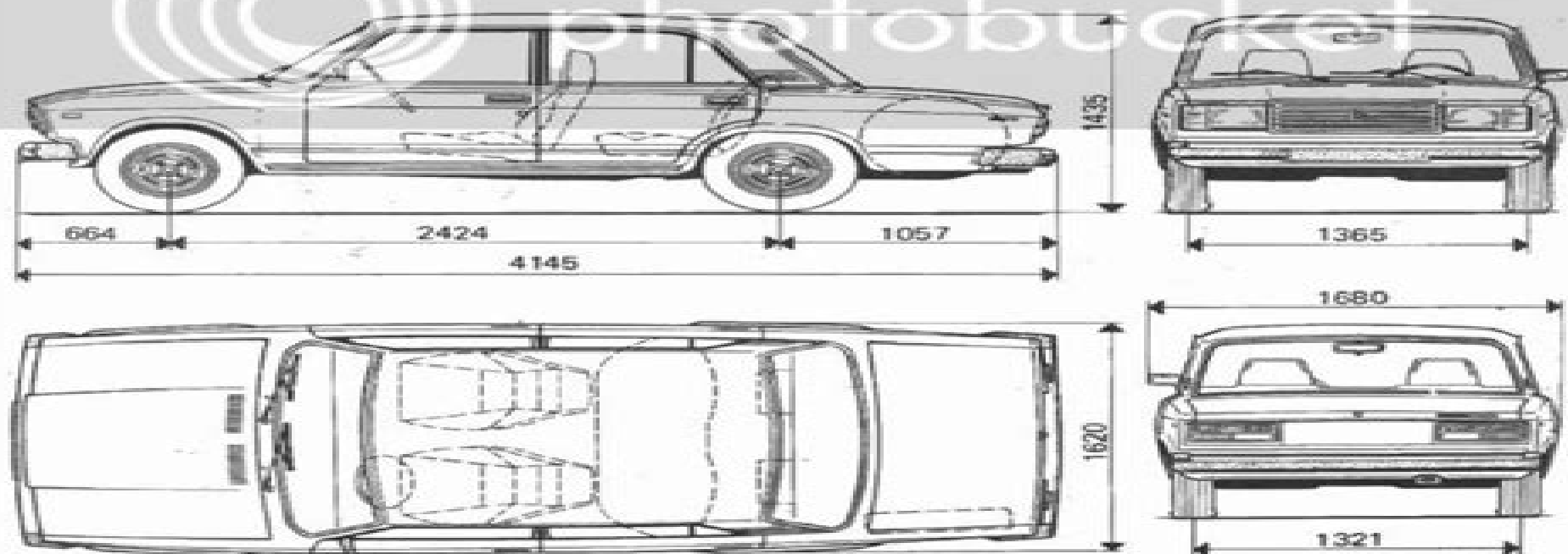
Fig. 1-1. Dimensiones principales del automóvil VAZ-2107
