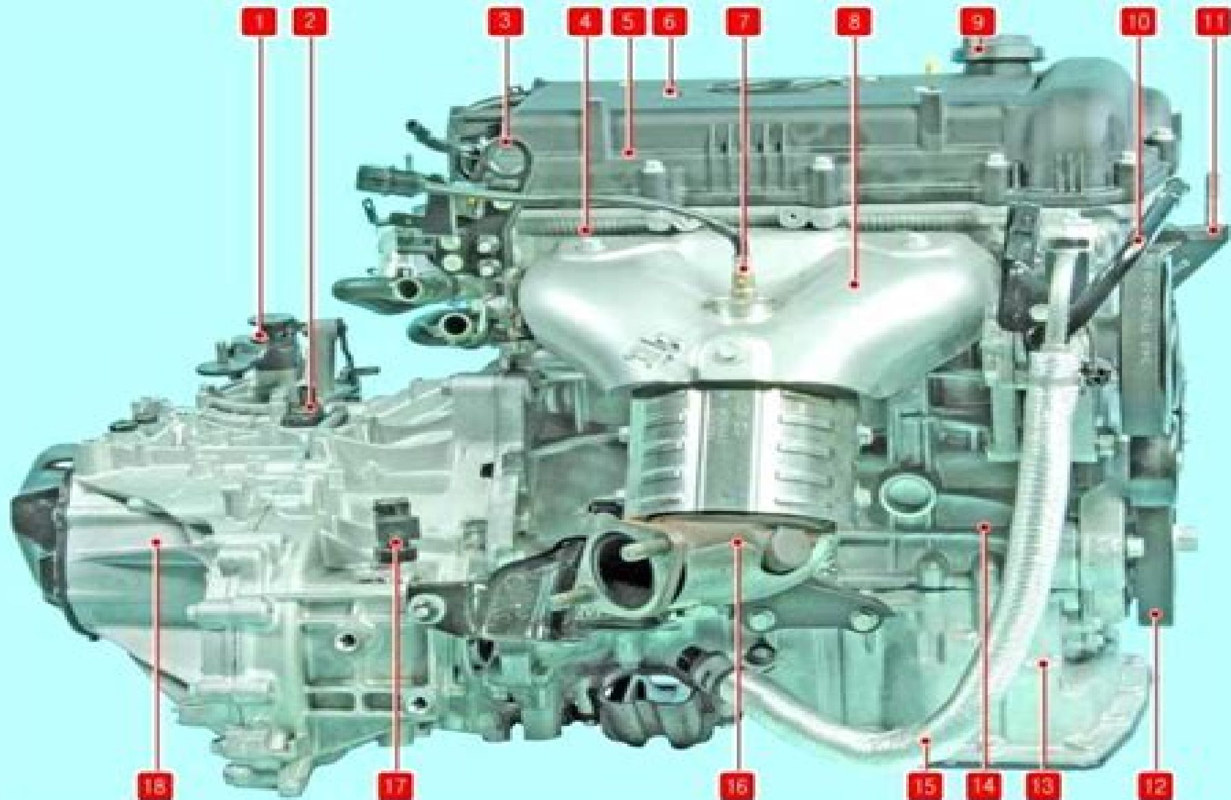
Двигатель (вид сзади): 1 – механизм переключения и выбора передач; 2 – выключатель света заднего хода; 3 – транспортный рым; 4 – головка блока цилиндров; 5 – крышка головки блока цилиндров; 6 – крышка свечных колодцев; 7 – управляющий датчик концентрации кислорода; 8 – термозащитный экран катколлектора; 9 – пробка масляной горловины; 10 – подающий трубопровод гидроусилителя рулевого управления; 11 – кронштейн крепления правой опоры подвески силового агрегата; 12 – ремень привода вспомогательных агрегатов; 13 – масляный картер; 14 – блок цилиндров; 15 – нагнетающий трубопровод гидроусилителя рулевого управления; 16 – катколлектор; 17 – датчик скорости автомобиля; 18 – коробка передач
