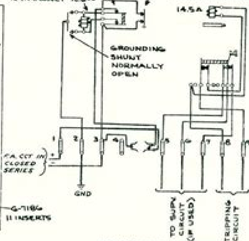
SCHEMATIC WIRING
