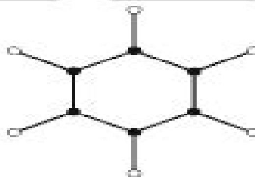
benzene
