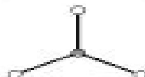
ammonia
