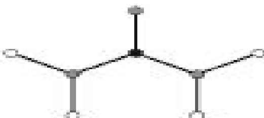
urea
