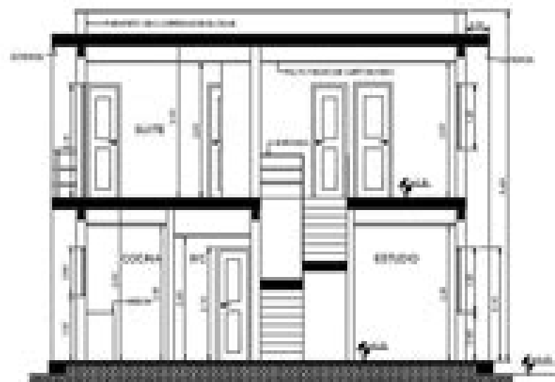
CORTE A-A'
