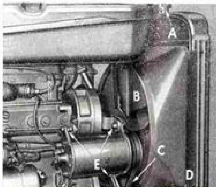
Fig. 29. Cooling System.
