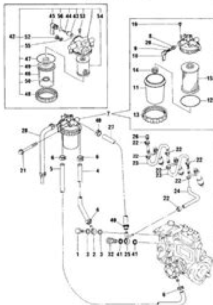
FIG. 5410 IMPIANTO COMBUSTIBILE FUEL LINE
