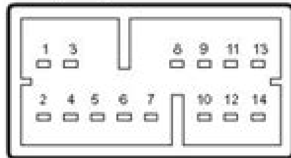
ET Connector(14P)
