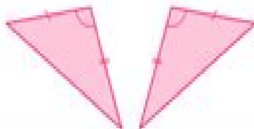
Side-angle-side (SAS)
