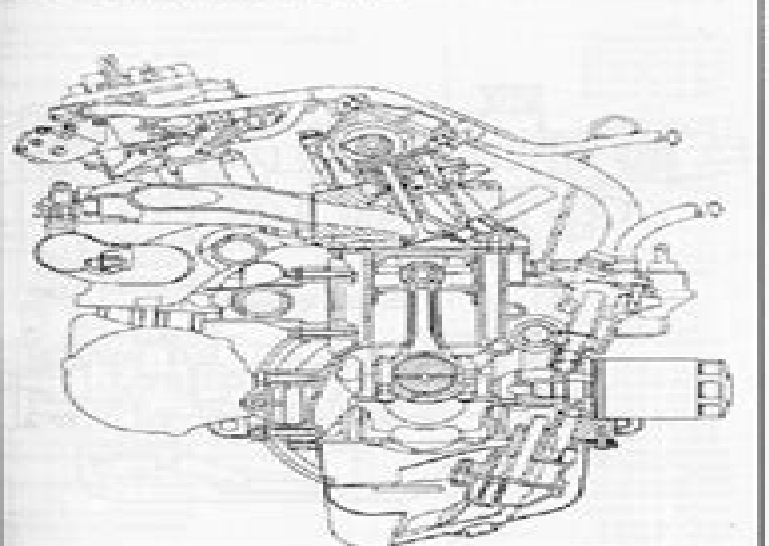
Fig. 26. Corte transversal del motor Tipo
