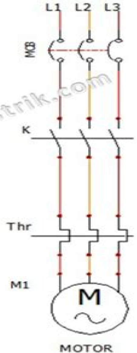
Rangkaian Utama
