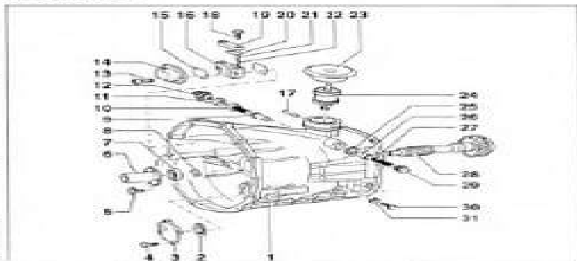
Рис. 5.24. Корпус сцепления, первичный вал и механизм переключения передач
