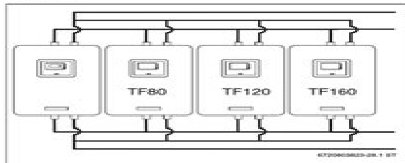
Bild 35 Stationen bauseits verbinden (hier: Anschlussseite rechts)
