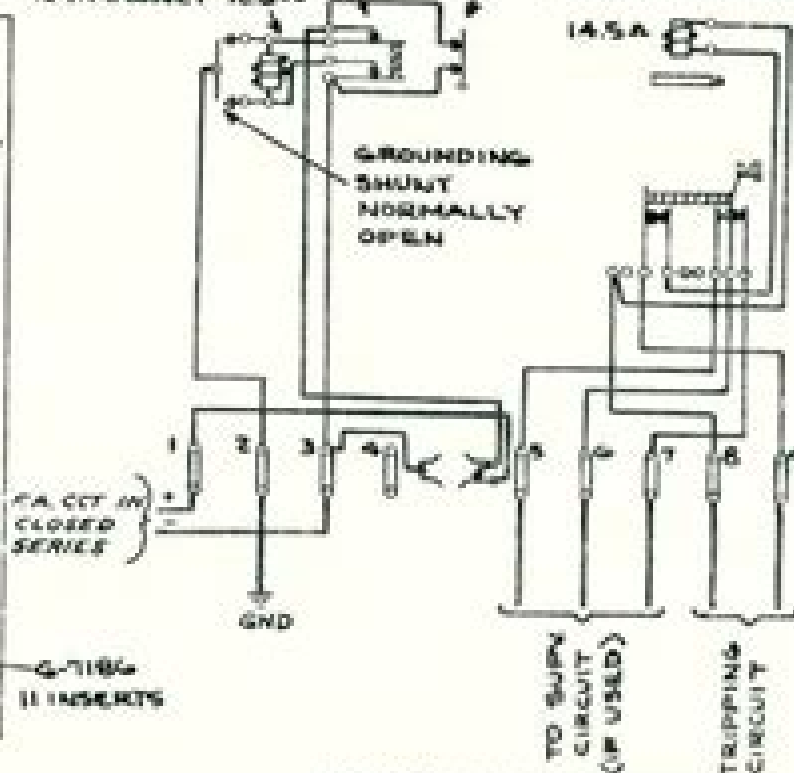
SCHEMATIC WIRING
