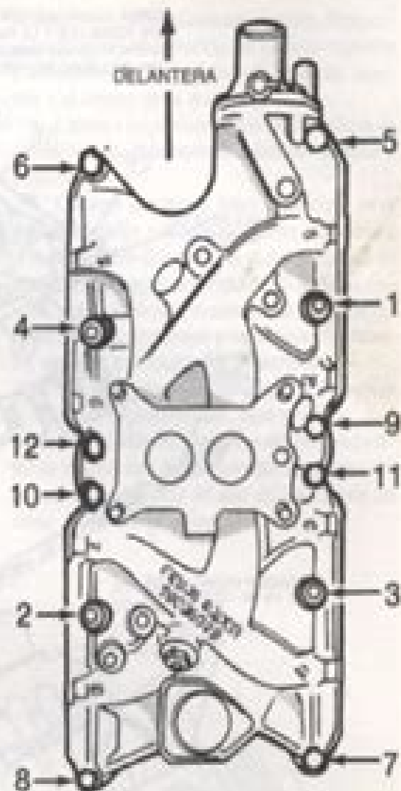
Secuencia de apriete de los tornillos del colector de admisión de los motores 8-255, 302 y 351W
