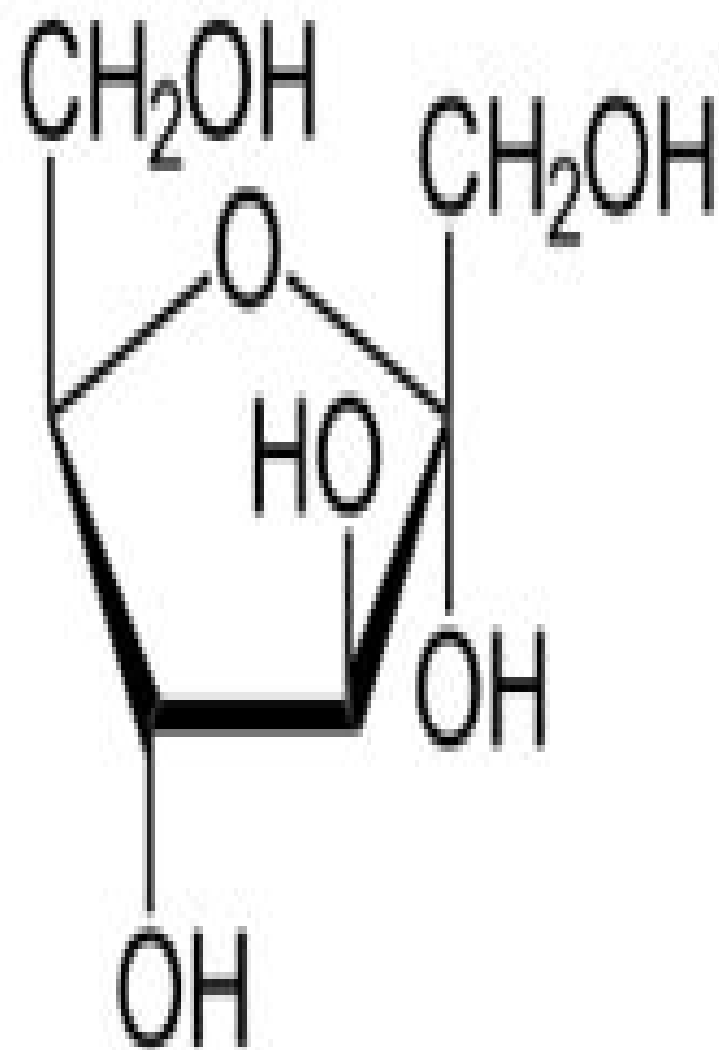
\alpha -D-Fructofuranose
