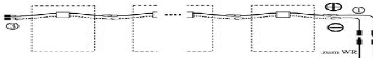
Abbildung 11: Prinzipzeichnung WR Anschluss RECHTE Dachseite: (Vorderansicht)
