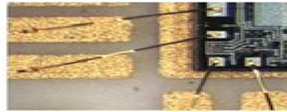
Wedgebonding
