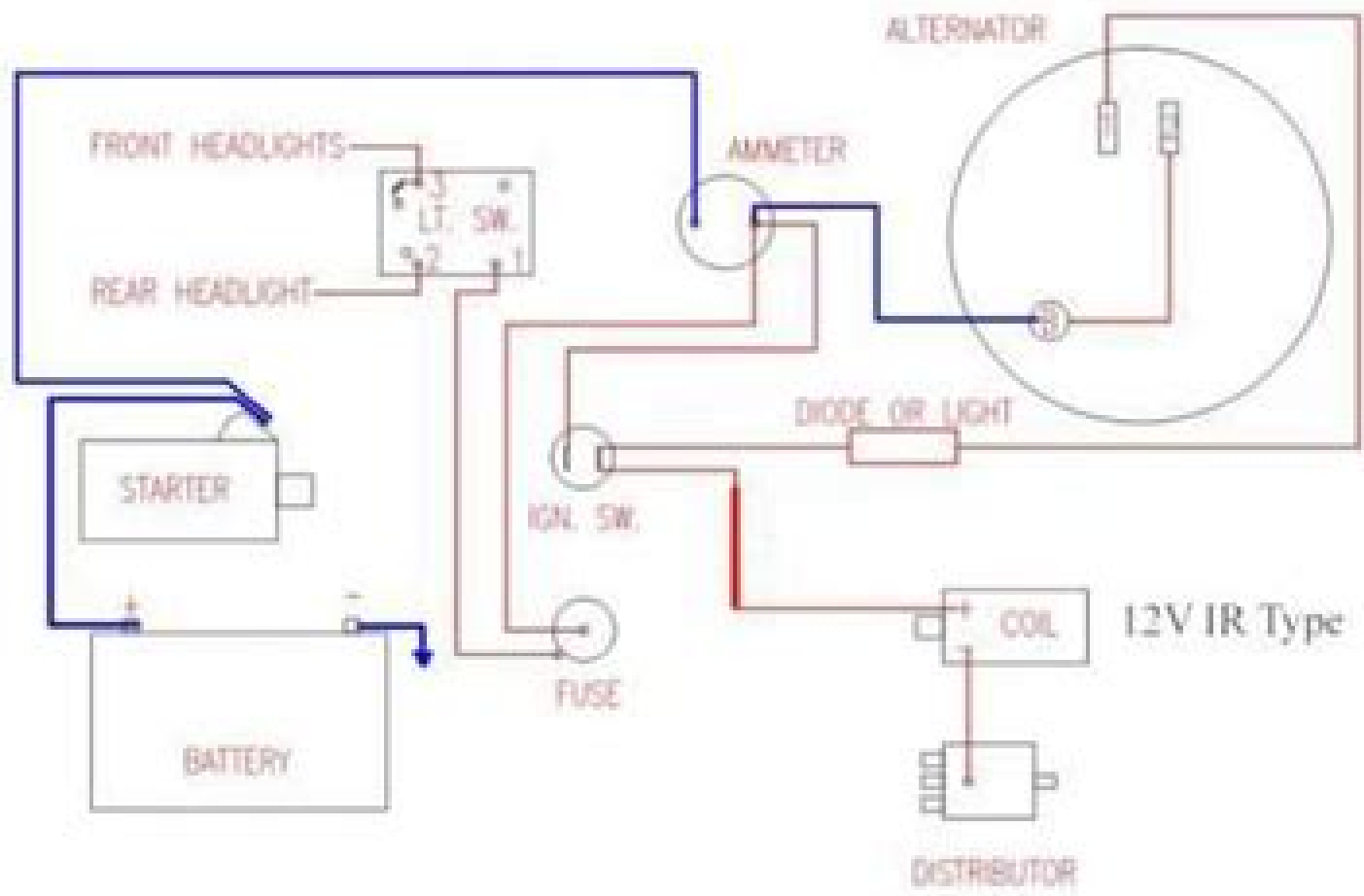
12 VOLT DIAGRAM
