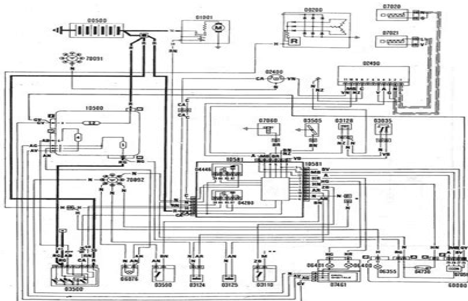
Рис. 11.36.4 Системы Digiplex и Citymatic, цифровые часы (модели ES с 1985г.)
