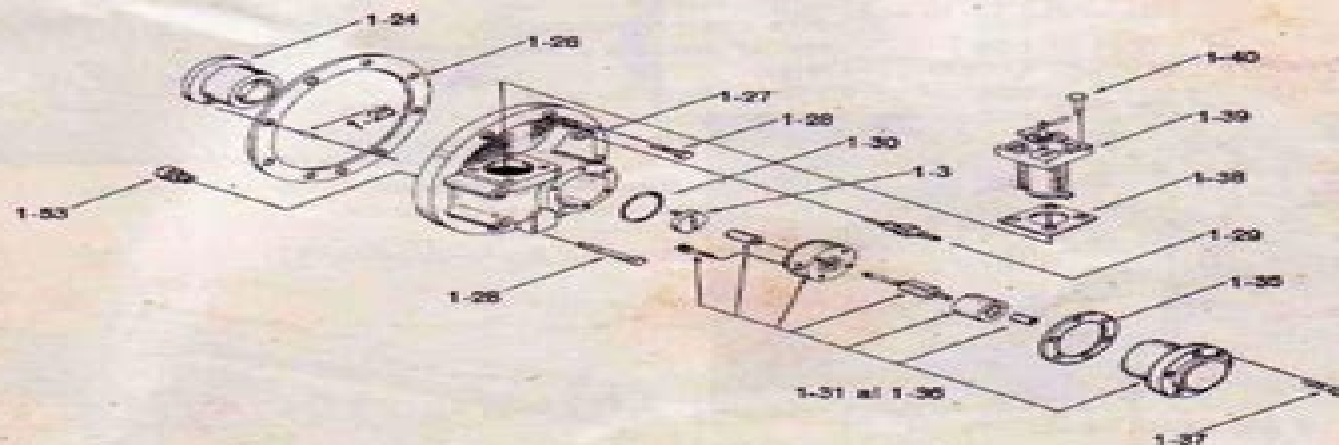
Fig. 63. Despiece de la sección cojinete lado bomba. Modelo A.
