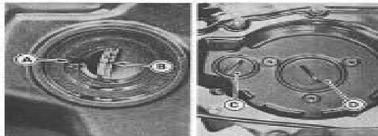
A. Slot B. T Mark
