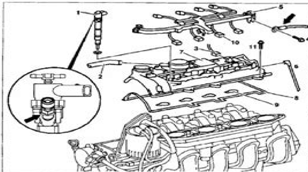
Рис. 2а. Снятие и установка крышки головки блока цилиндров на двигателях 611.981/983/987:
