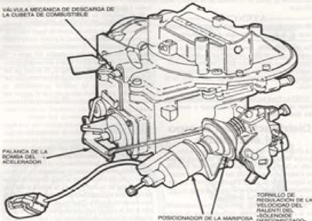
Carburador para motor 2150, con solenoide
