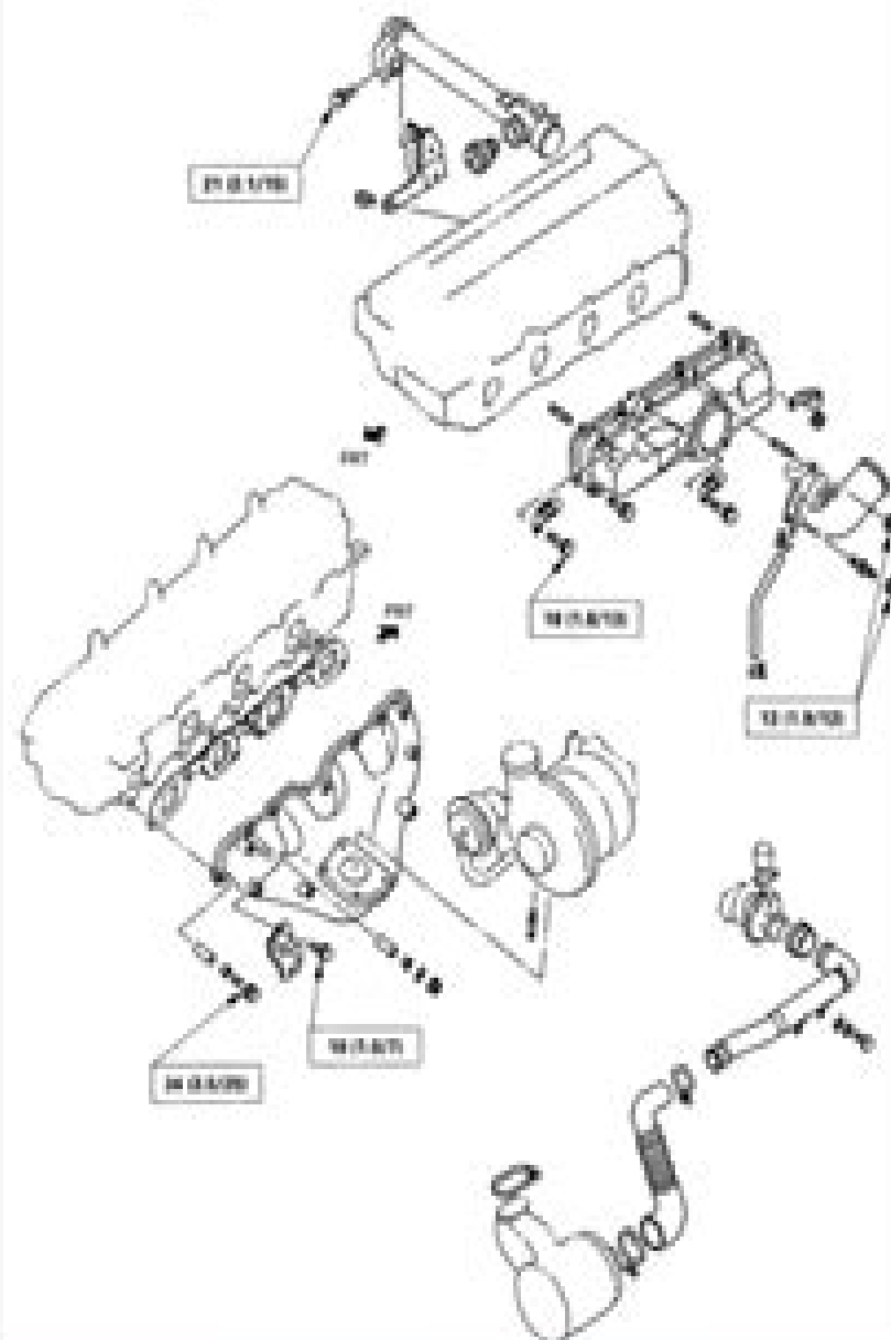
4HE1-T / 4HE1-TC Engine
