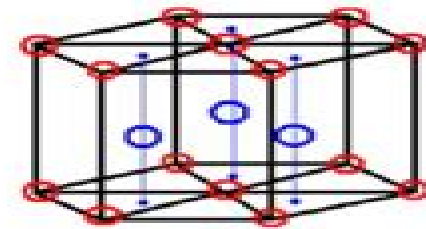
HCP
