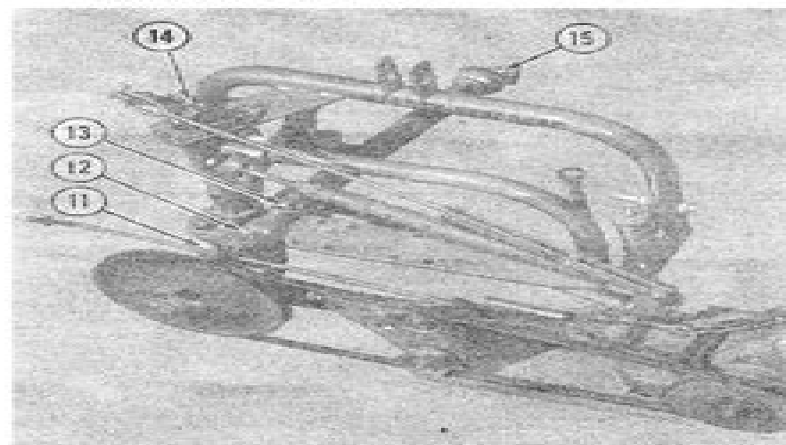
Fig. 2 - Lubrication Points
