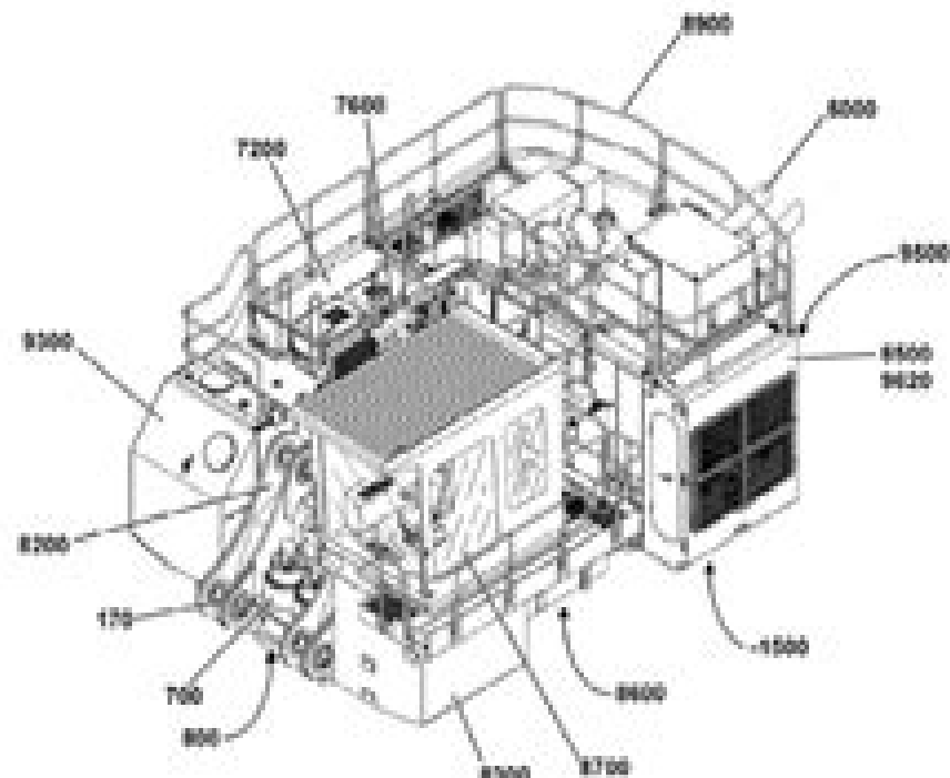
Fig. 1-1 Uppercarriage
