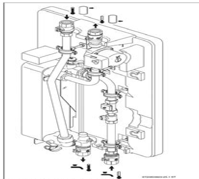
Bild 36 Anschlussbelegung Einzelstation
