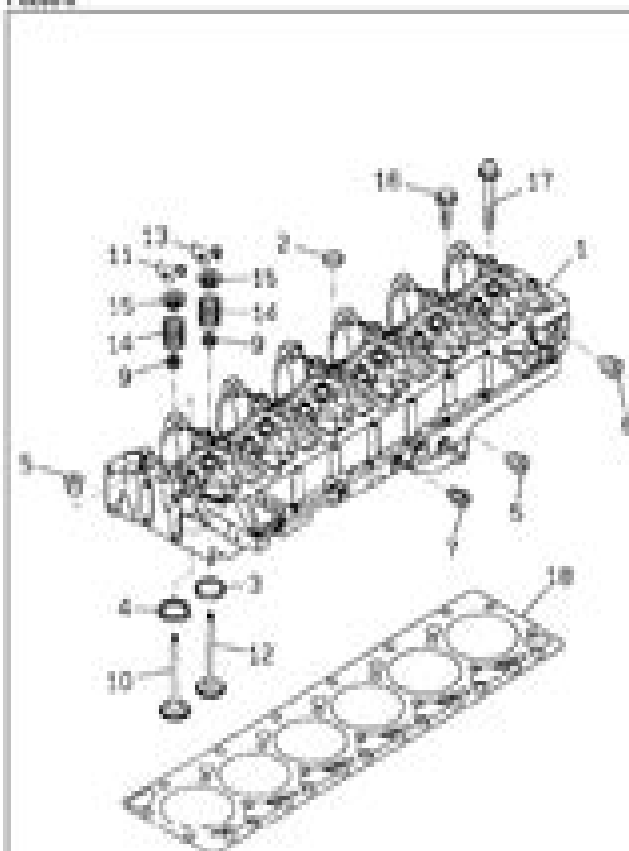
PC200-6
