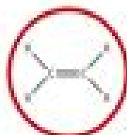
ALKENE
