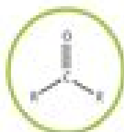
KETONE
