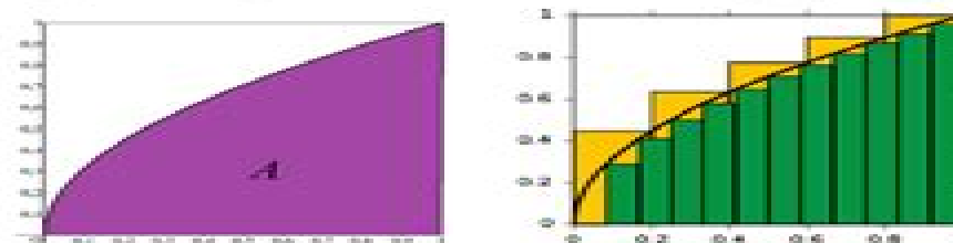
La región A y las sumas de Riemann para n = 5 y n = 12 .
