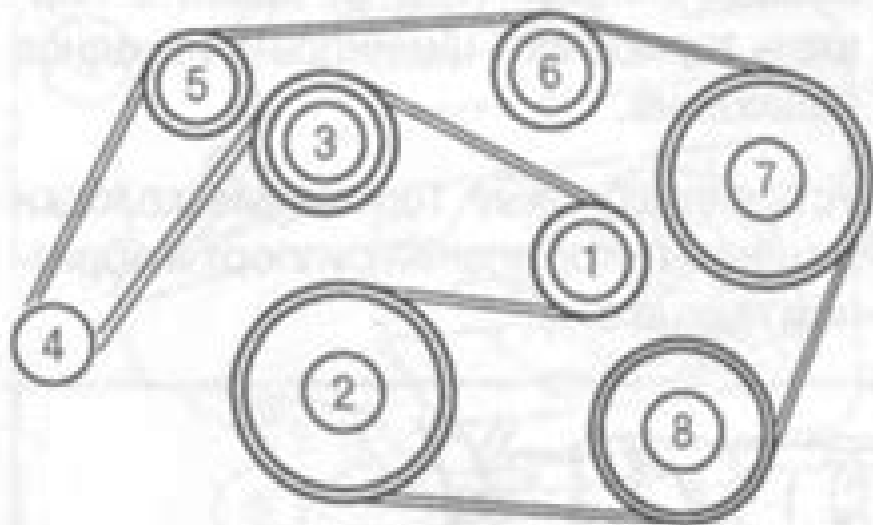
Схема установки ремня привода вспомогательных механизмов для автомобилей с кондиционером
