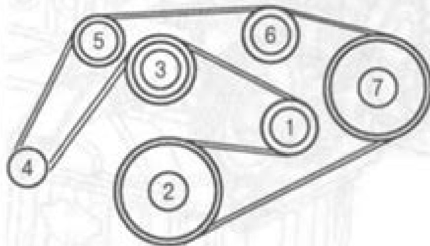
Схема установки ремня привода вспомогательных механизмов для автомобилей без кондиционера
