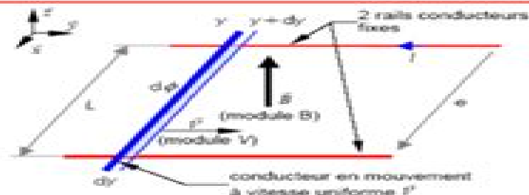
Figure 1 : barre en translation dans le champ B .
