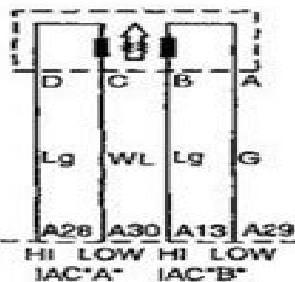
Клапан управления холостым ходом
