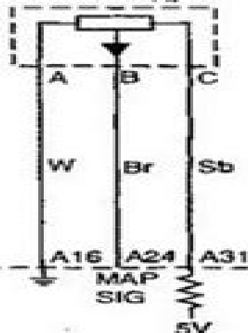
Блок управления двигателем HV - 240
