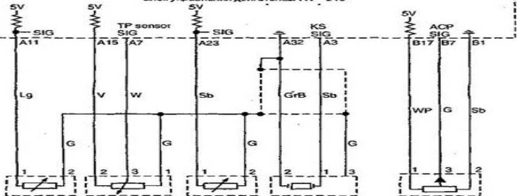
Датчик температуры охлаждающей жидкости
