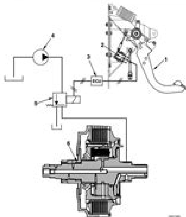
Fig. 11 - Main clutch actuation
