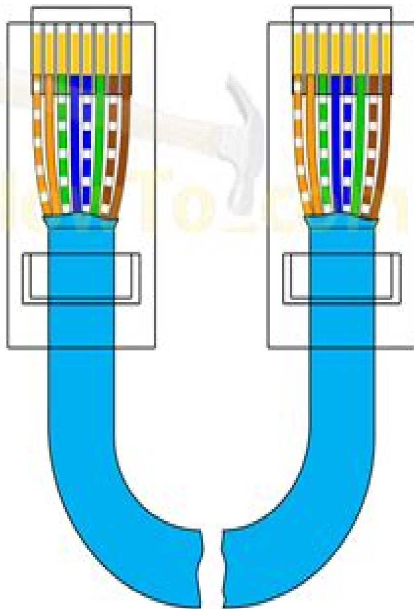
EIA/TIA T568B
