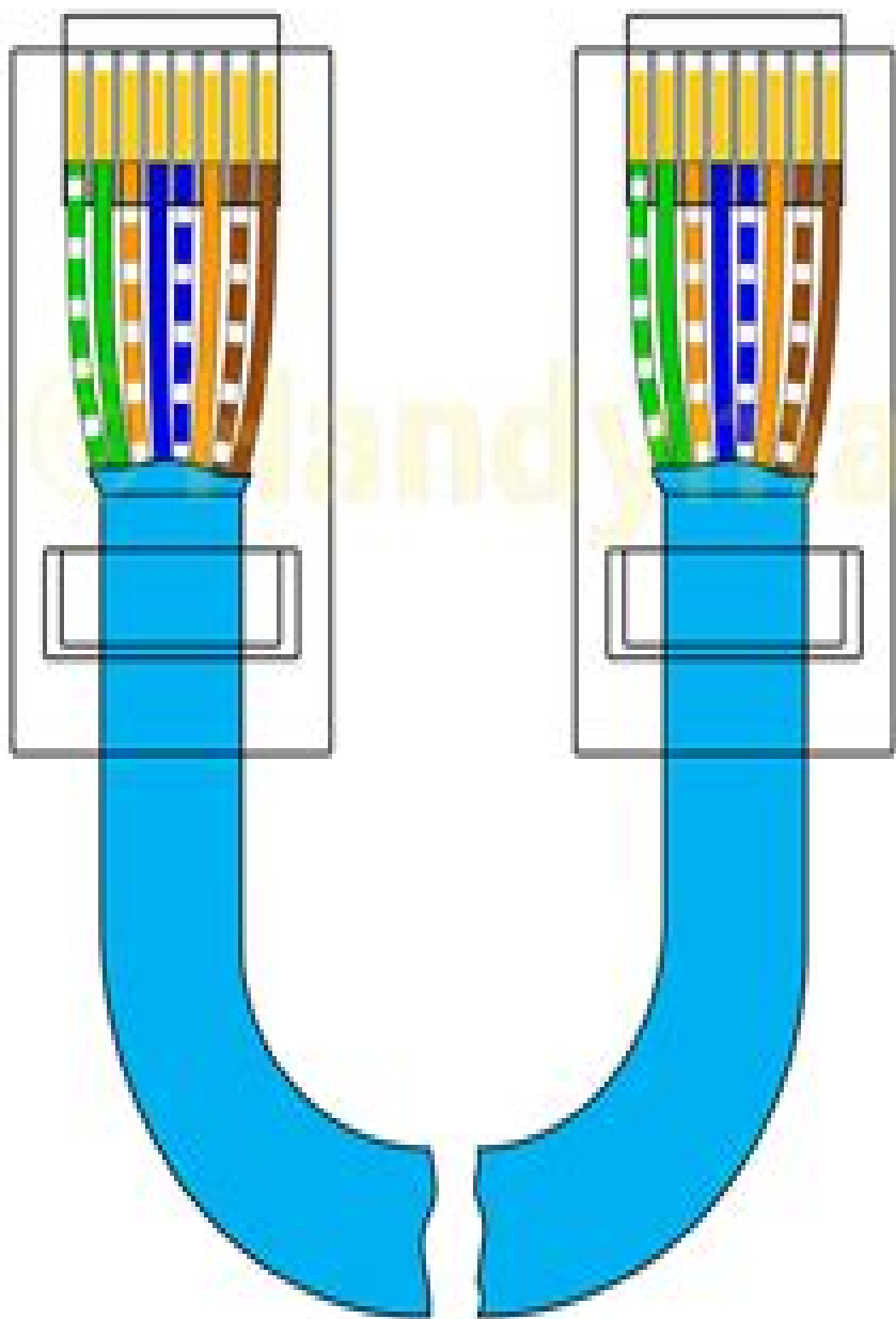
EIA/TIA T568A
