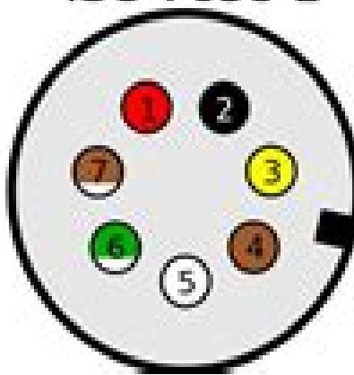
ISO 7638-2
