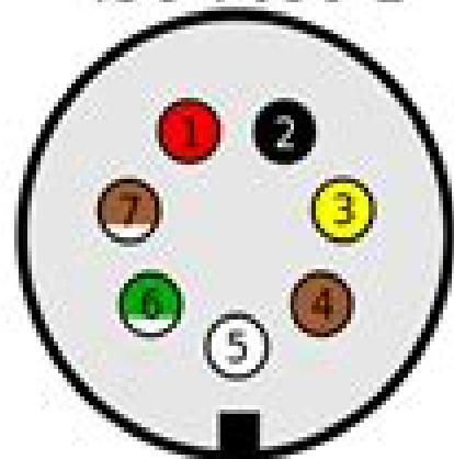
ISO 7638-1
