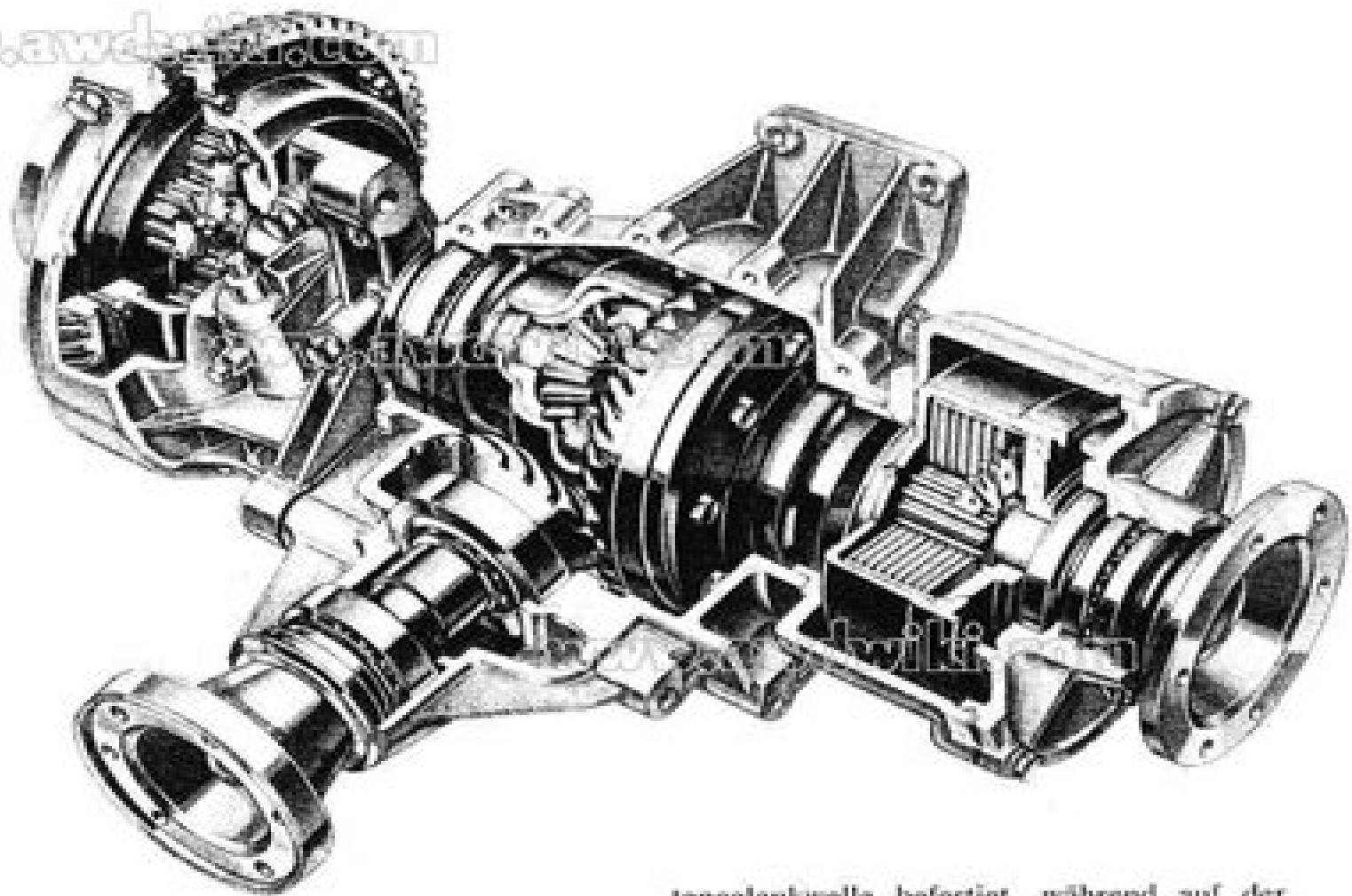
Bild 5.23 Vorderachs-Aggregat des Lancia Delta HF 4WD zur Antriebsverzweigung. Am Planeten-Mittendifferential wird die linke Sei-
