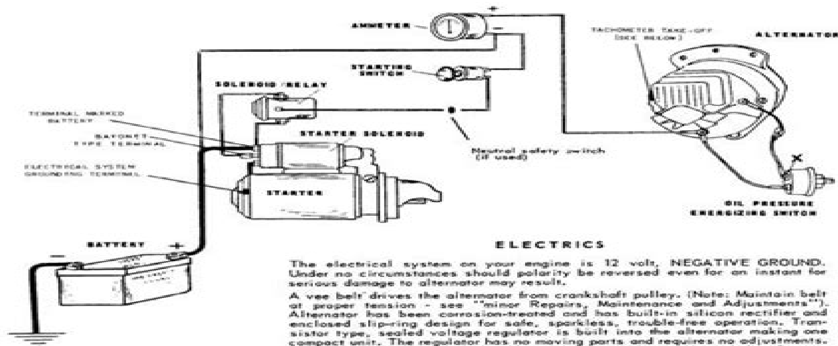
FIG. 15 WIRING DIAGRAM
