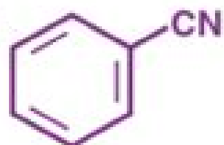
Benzonitrile
