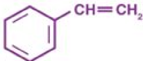
Styrene
