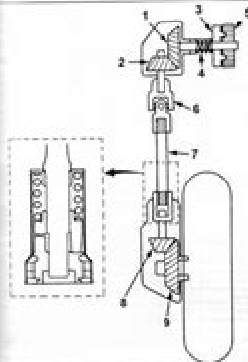
Principio de transmisión secundaria por cardán. 1. Piñón del par cónico de salida de caja - 2. Piñón conducido de par cónico - 3. Leva de amortiguador - 4. Muelle - 5. Piñón receptor del eje del piñón de ataque - 6. Cardán - 7. Eje de transmisión - 8. Piñón de ataque del par cónico trasero - 9. Corona de par cónico trasero.
